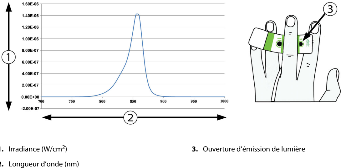
Figure A-1 : Irradiance spectrale et emplacement de l'ouverture d'émission de lumière
