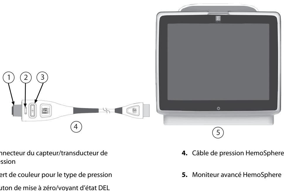
Figure 4-2 : Description du raccordement du câble de pression
