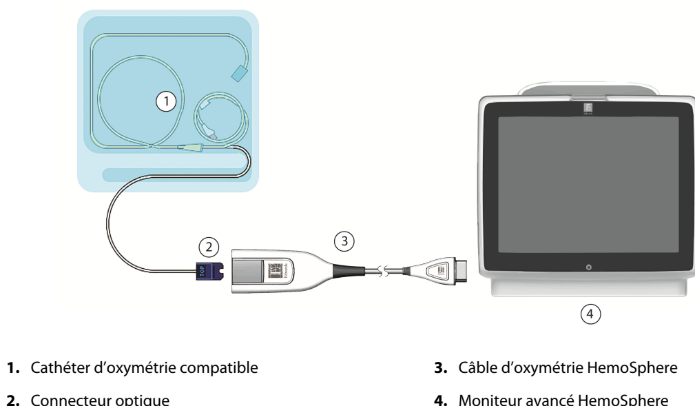
Figure 4-3 : Présentation des connexions d'oxymétrie
