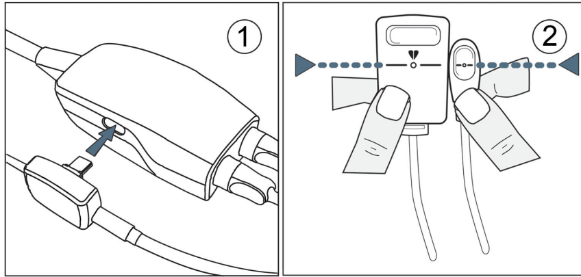
Şekil 11-7: Kalp referans sensörü kalibrasyonu
