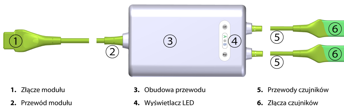
Rysunek 13-1: Przewód do oksymetrii ForeSight — widok z przodu
