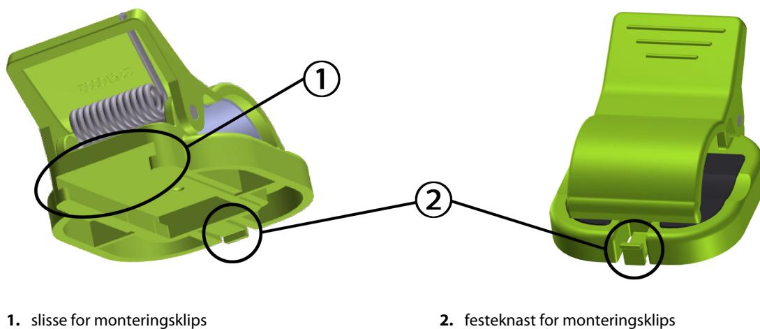
Figur 13-3: Festepunkter for monteringsklips
