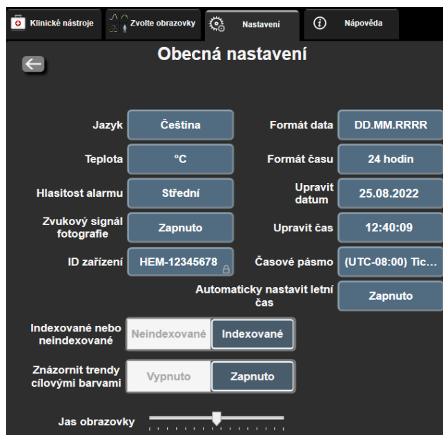
Obrázek 6-3: Obecná nastavení monitoru
