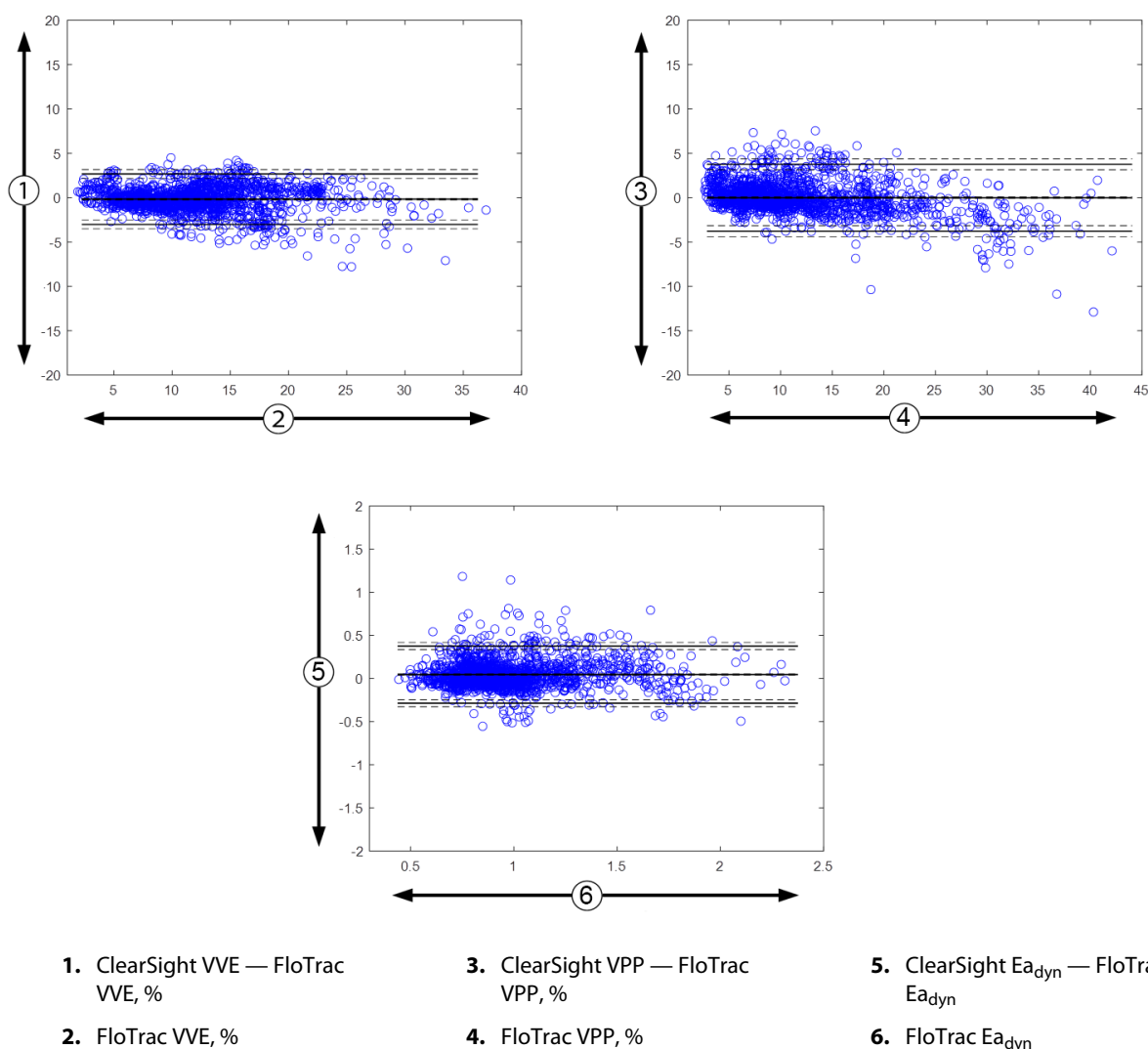
Figure 14-8 : Graphiques de Bland-Altman pour les paramètres VVE, VPP et Ea_{dyn}
