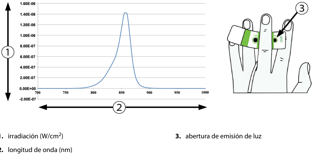
Figura A-1: Irradiación espectral y localización de la abertura de emisión de luz
