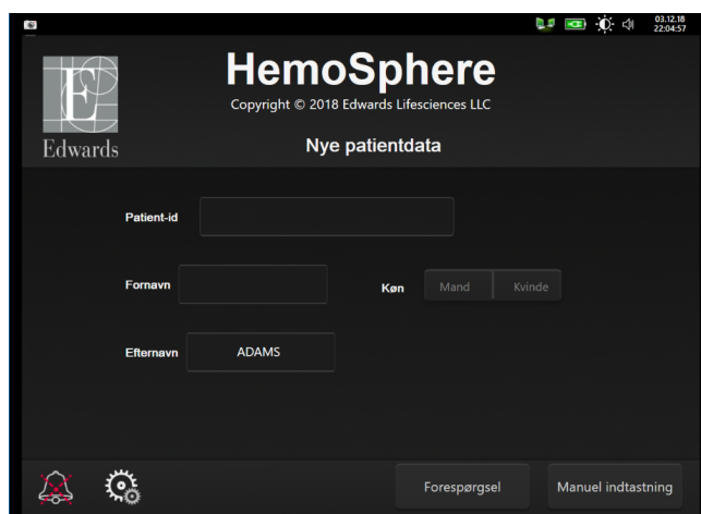
Figur 8-1: HIS-patientforespørgselsskærm
