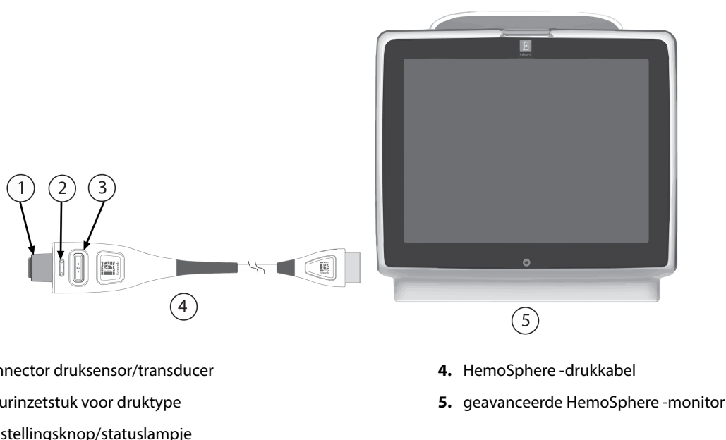
Afbeelding 4-2: Overzicht drukkabelaansluitingen
