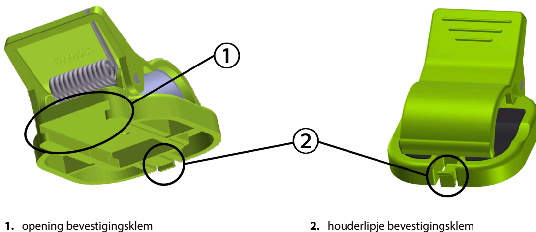
Afbeelding 13-3: Bevestigingspunten bevestigingsklem
