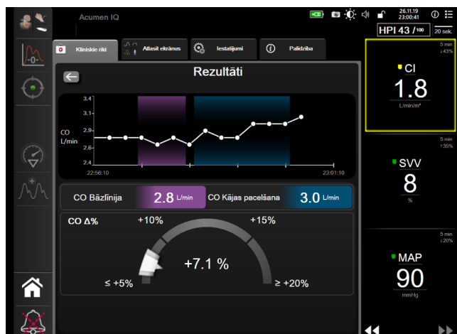
14-14. attēls. Šķidruma reakcijas tests — ekrāns Rezultāti
