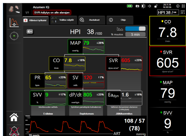
Kuva 14-6: Toinen HPI-näyttö
