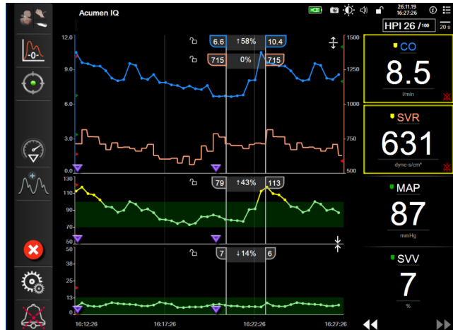
Kuva 5-7: Trendikuvaajanäyttö
