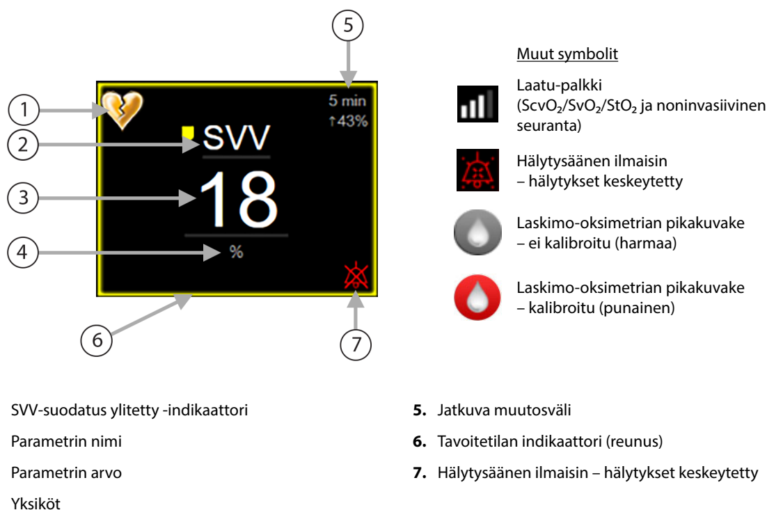
Kuva 5-5: Parametriruutu
