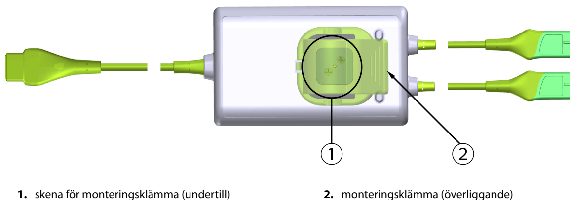
Figur 13-2: Vy bakifrån för FORE-SIGHT ELITE -oximetrimodul
