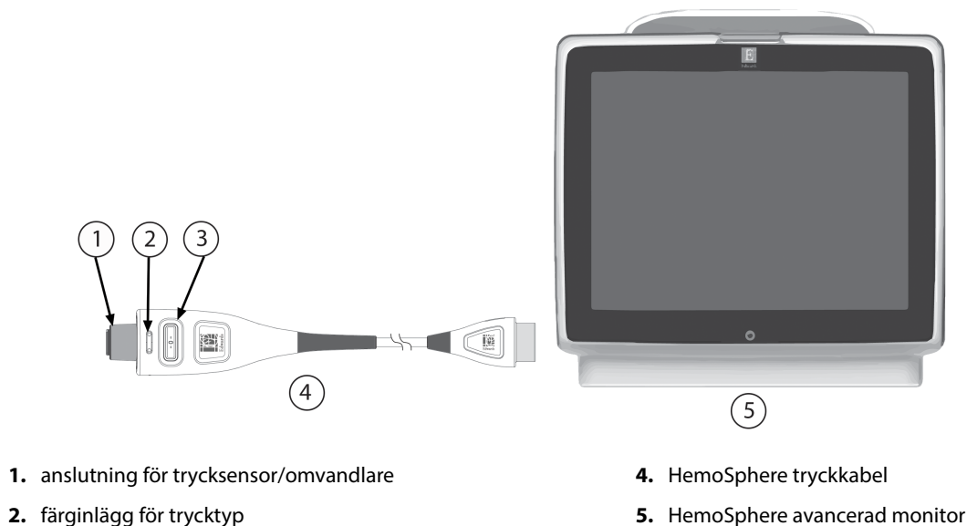
Figur 4-2: Översikt över tryckkabelanslutning
