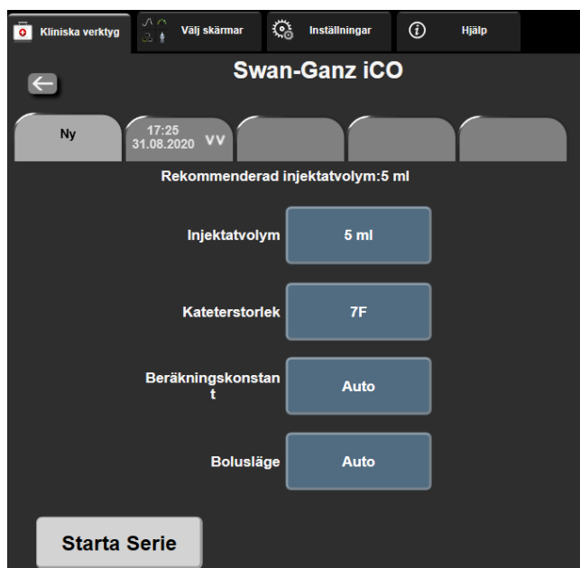
Figur 9-6: Konfigureringskärmen iCO ny inställning
