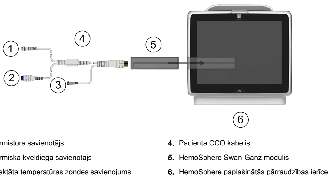
4-1. attēls. HemoSphere Swan-Ganz moduļa monitoringa savienojumu pārskats
