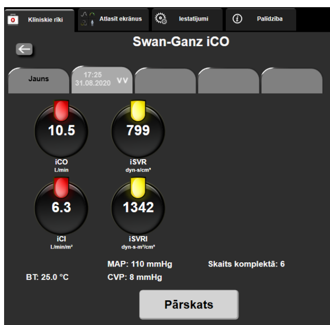
9-7. attēls. Termodilūcijas kopsavilkuma ekrāns
