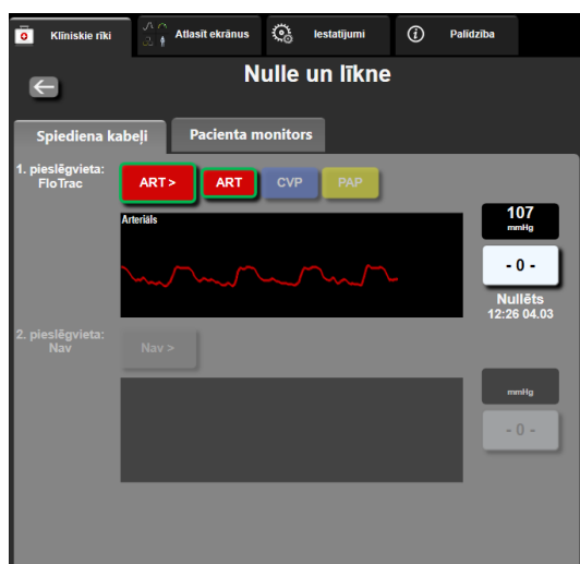
10-2. attēls. Nulles un līkņu ekrāni — nulles sensors un spiediena izvade
