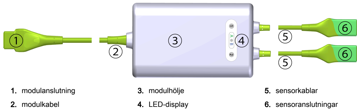
Figur 13-1: Vy framifrån för FORE-SIGHT ELITE -oximetrимodul
