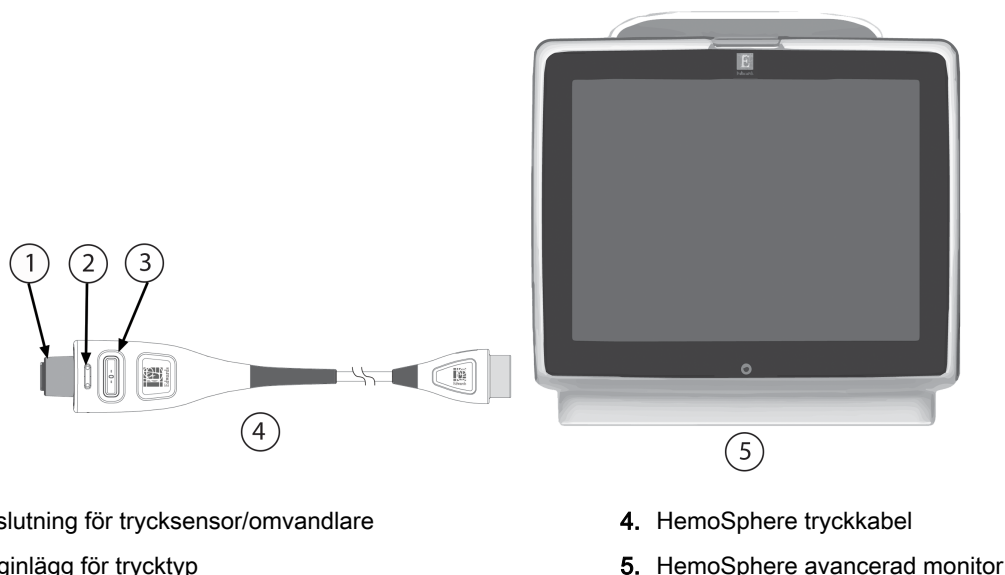
Figur 4-2: Översikt över tryckkabelanslutning
