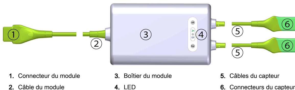
Figure 13-1 : Vue avant du module d'oxymétrie FORE-SIGHT ELITE
