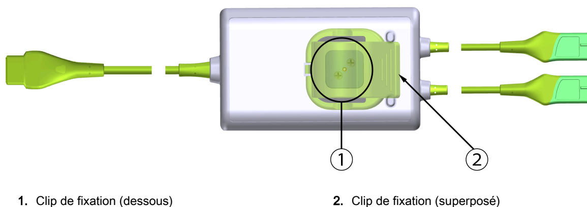
Figure 13-2 : Vue arrière du module d'oxymétrie FORE-SIGHT ELITE
