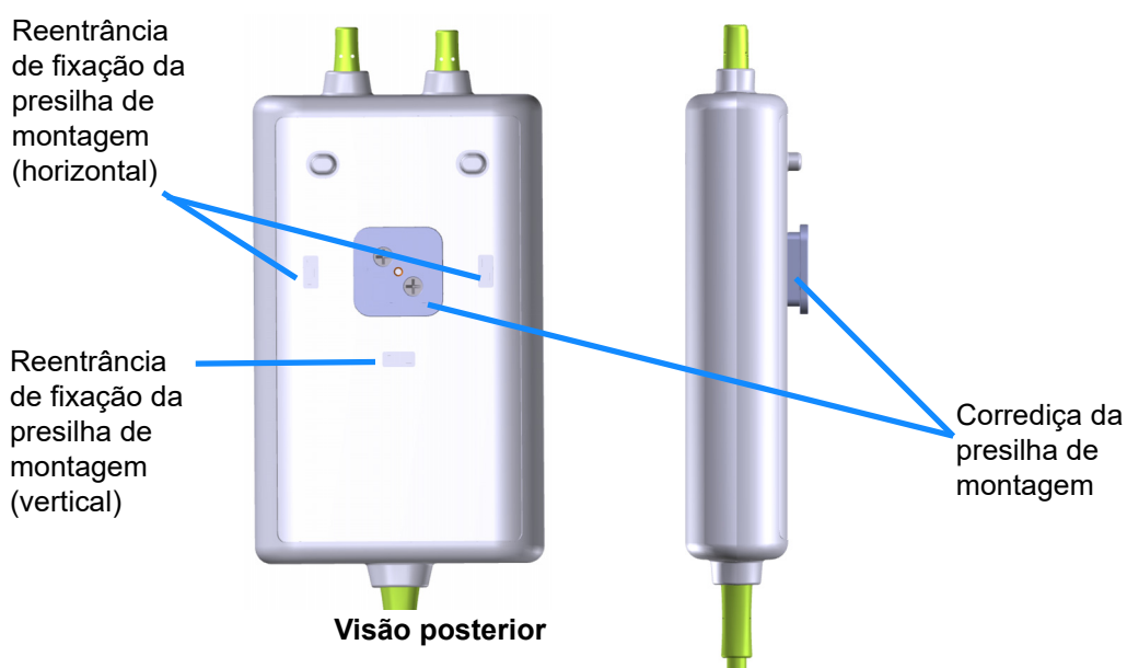
Figura 12-4 Estojo do módulo – pontos de encaixe da presilha de montagem
