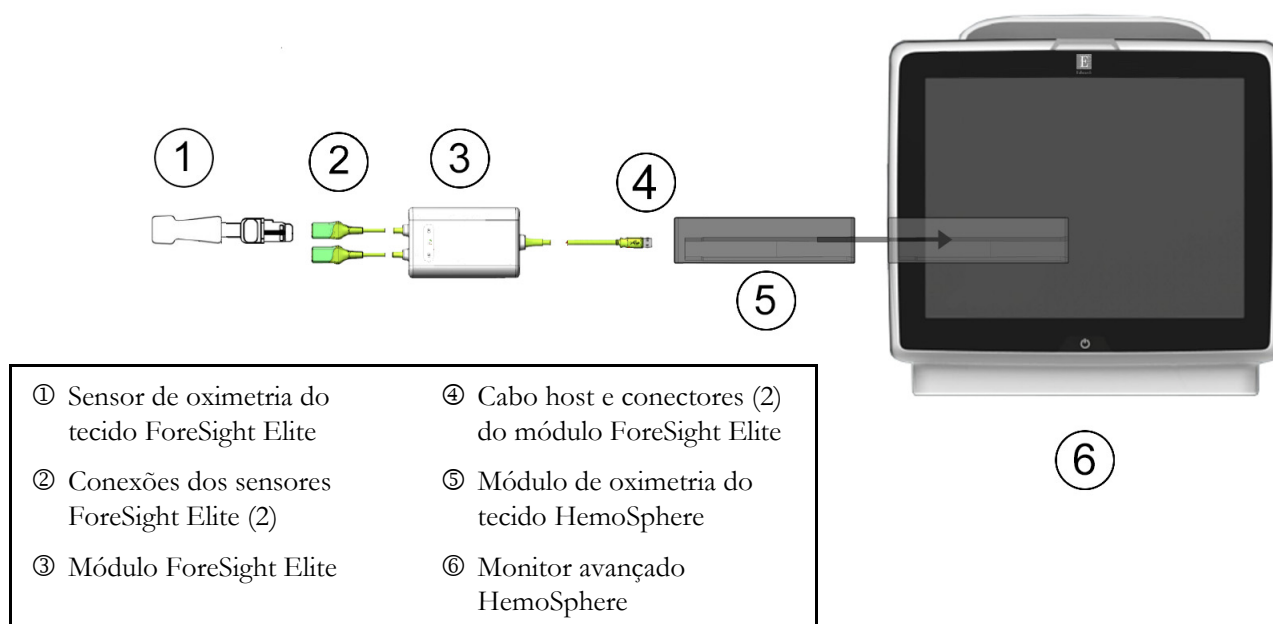
Figura 12-8 Visão geral da conexão do módulo de oximetria do tecido HemoSphere
