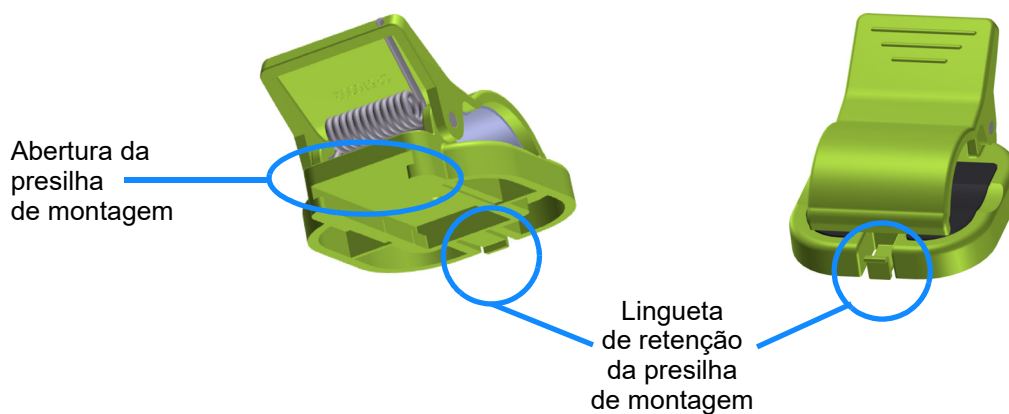
Figura 12-3 Presilha de montagem – pontos de encaixe da corredeira do módulo
