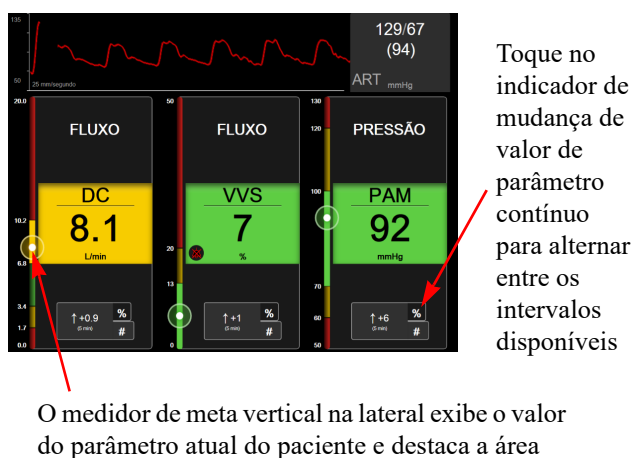
Figura 5-21 Tela principal focalizada
