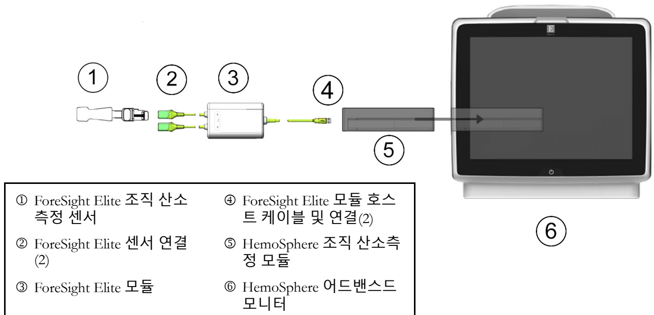
그림 12-8 HemoSphere 조직 산소측정 모듈 연결 개요
