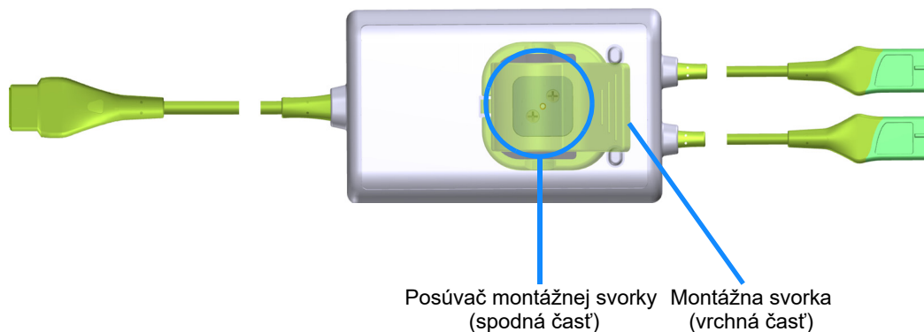
Obrázok 12-2 Tkanivový oxymeter ForeSight Elite – pohľad zozadu
