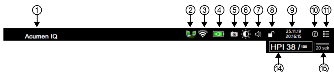
Figur 5-26 Informasjonslinje – HemoSphere-trykkabel
